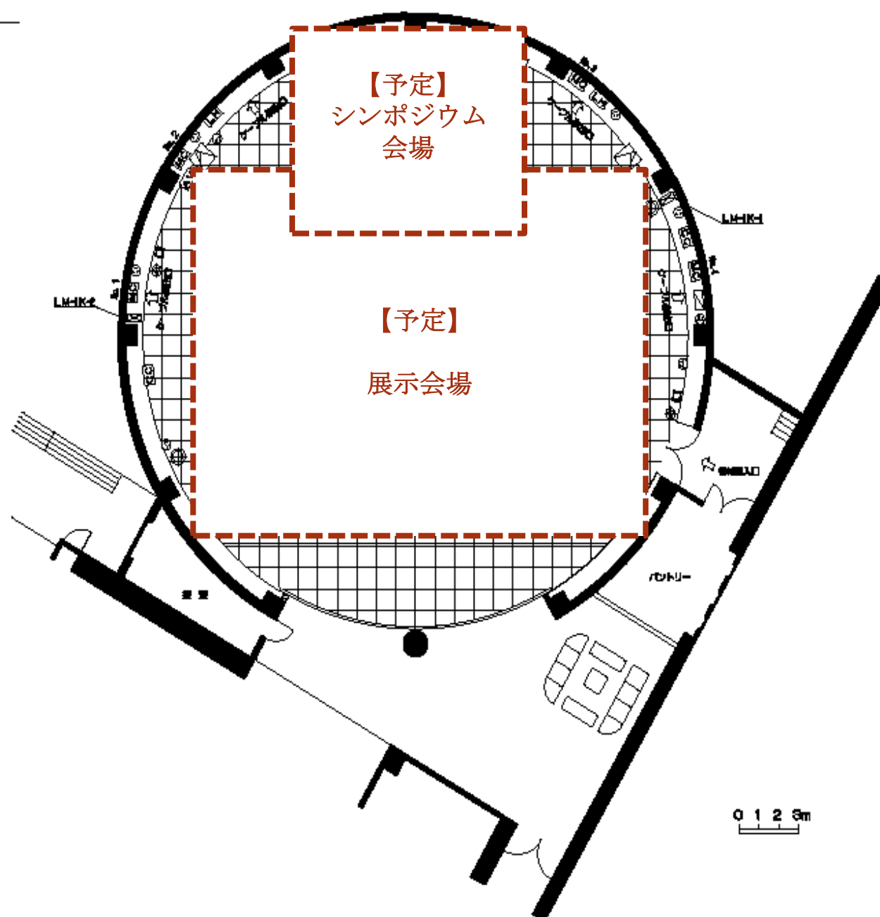
多目的ホール平面図 S=1:200
